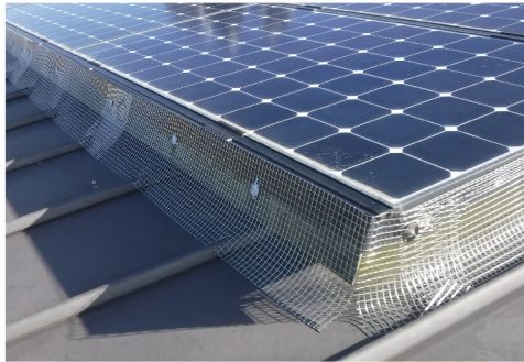
ハト侵入防止用ステンレス製網 取付施工
